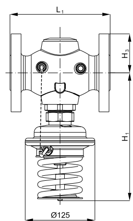
AVD D y 32–50 P рег = 1–5 бар
