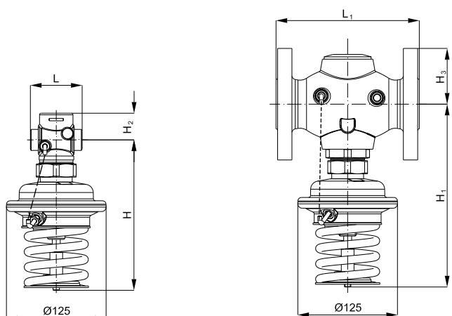
AVD D y 15–25 P рег = 1–5 бар
